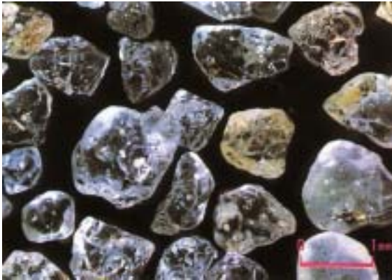
【石英】 石英の結晶を水晶と呼びます
